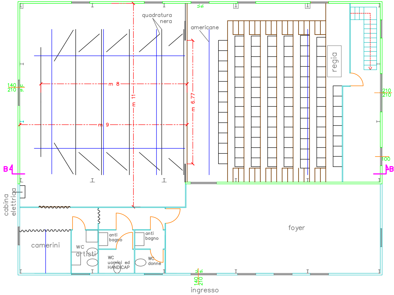
PIANTA Scala 1:100
